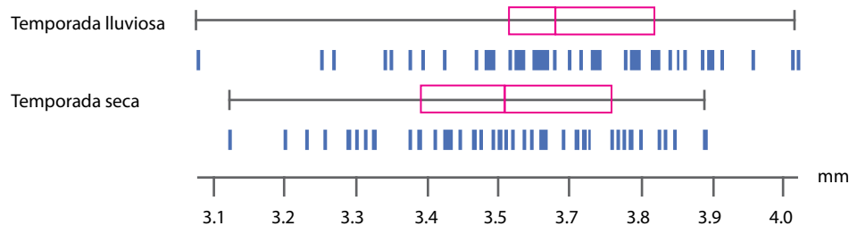
Figura 3. Análisis de tamaño centroide alar. Muestra la variación en el tamaño centroide en milímetros (mm) de las alas, en las temporadas seca y lluviosa. Las líneas verticales azules representan especímenes. Las cajas muestran la media como una línea vertical central junto con los percentiles 25 y 75 a ambos lados
