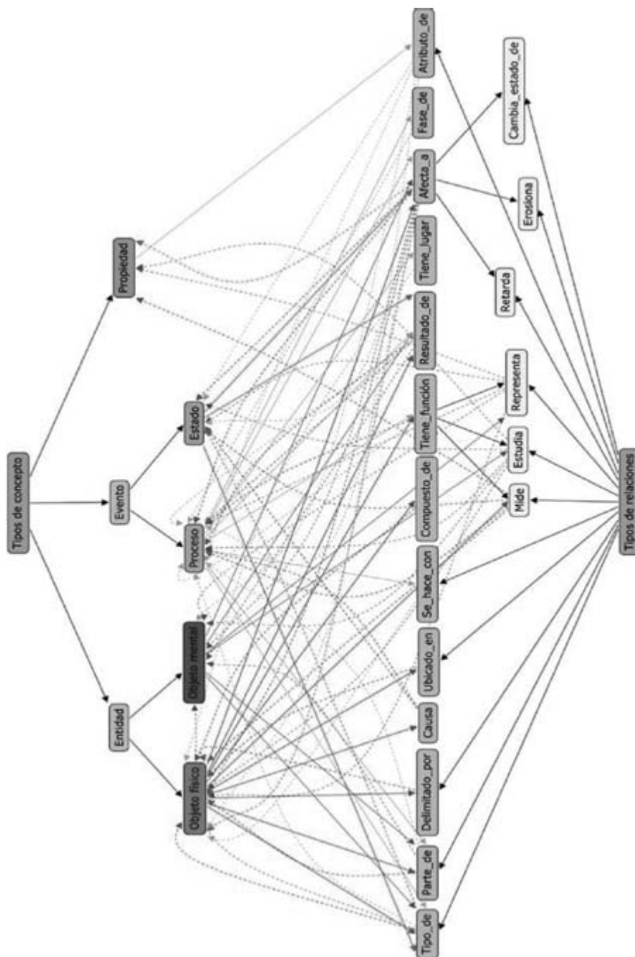
Figura 4 Interdependencia concepto-relación-concepto
