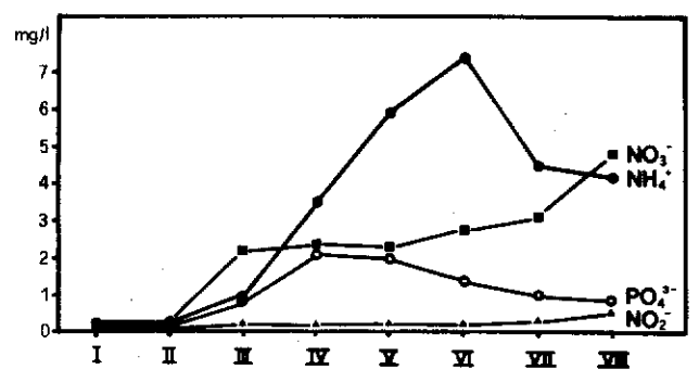
Fig. 7: Valores promedio para amonio, nitrato, nitrito y fosfato a lo largo del río Medellín.
