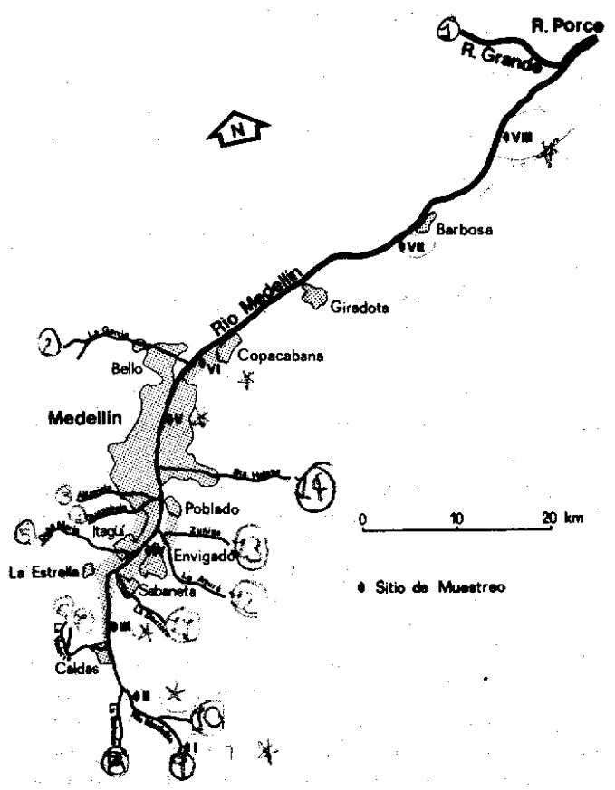
Fig. 1: Esquema de la hoya hidrográfica del río Medellín y sus principales afluentes.
