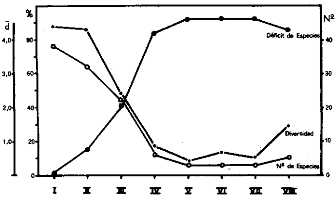
Fig. 9: Diversidad, número y déficit de especies a lo largo del río Medellín.
