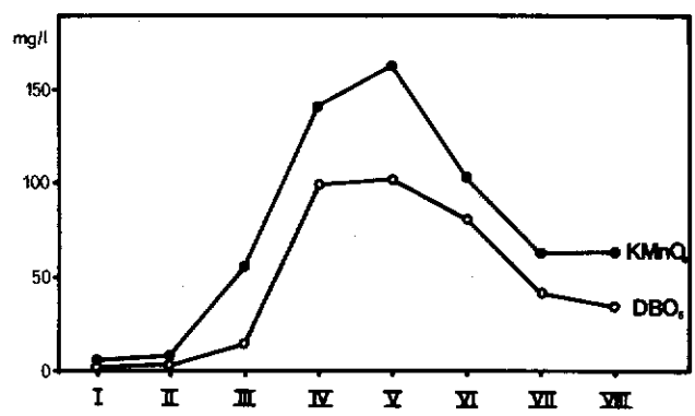
Fig. 6: Valores promedio de la DBO5 y la demanda de KMnO4 a lo largo del río Medellín.
