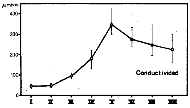
Fig. 5: Valores promedio de conductividad a lo largo del río Medellín. (Las barras verticales indican valores máximos y mínimos).
