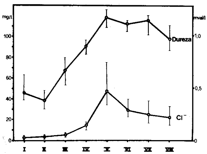
Fig. 8: Valores promedio de dureza y cloruro a lo largo del río Medellín. (Las barras verticales indican valores máximos y mínimos).
